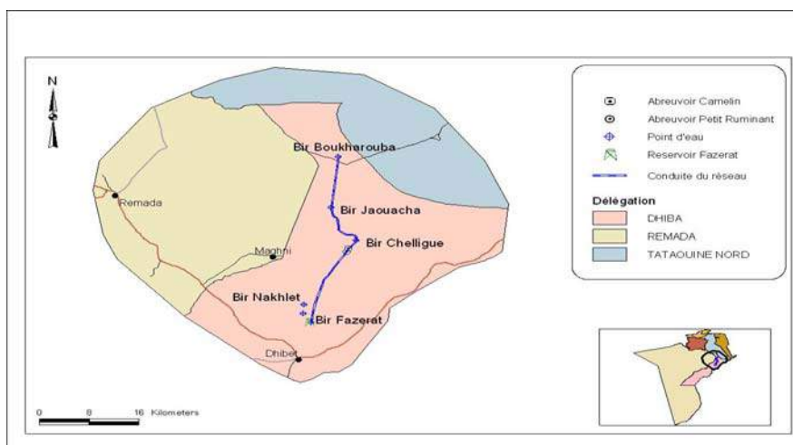
Figure n° 2 : Circuit d'acheminement de l'eau pastorale du réseau Fazrat dans les parcours collectifs d'El Ouara (d'après Ben Saad, 2002)
